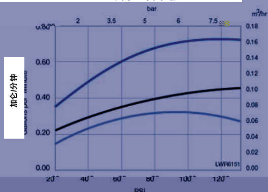
射流器“J”（浅蓝色） 用于10英寸罐
