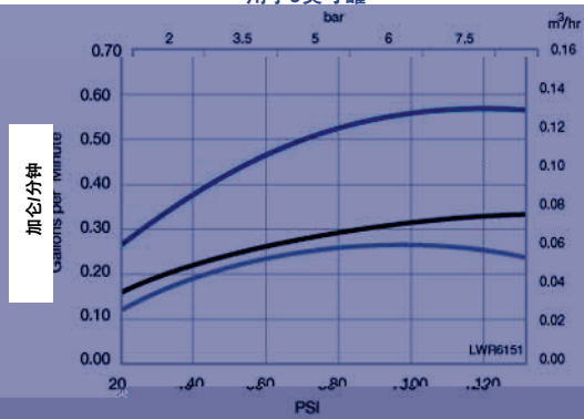
射流器“H”（浅紫色） 用于9英寸罐
